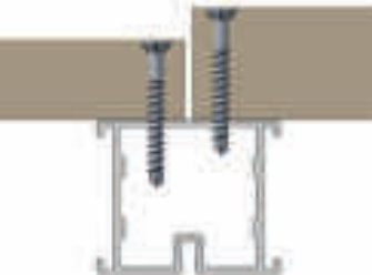
Speedfix Schraube 5,5 x 45 mm / 5,5 x 60 mm A4.
