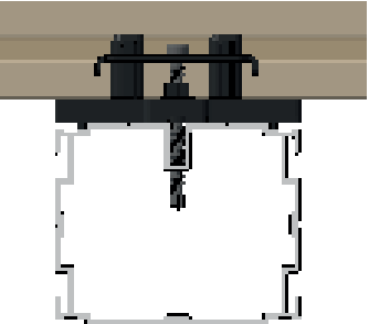
BS 4,2 X 38 EDELSTAHL A2 SCHWARZ
