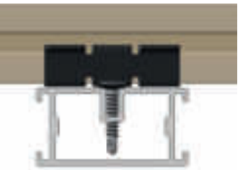
BS 3,9 X 22 EDELSTAHL A2
